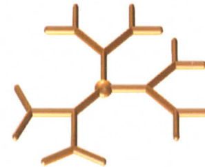
Dendrimer
